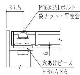
ボルト固定部詳細
