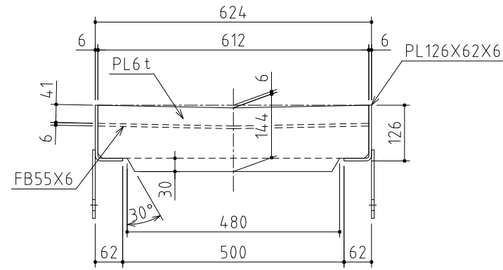
A-A 矢視図
