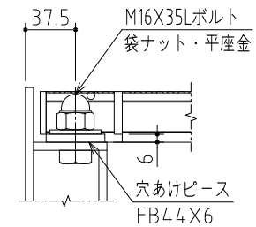
ボルト固定部詳細
