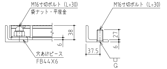
ボルト固定部詳細
