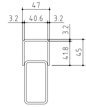
A部詳細
