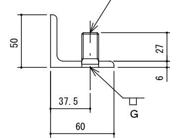
寸切ボルト部詳細図
