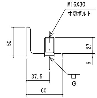
寸切ボルト部詳細図
