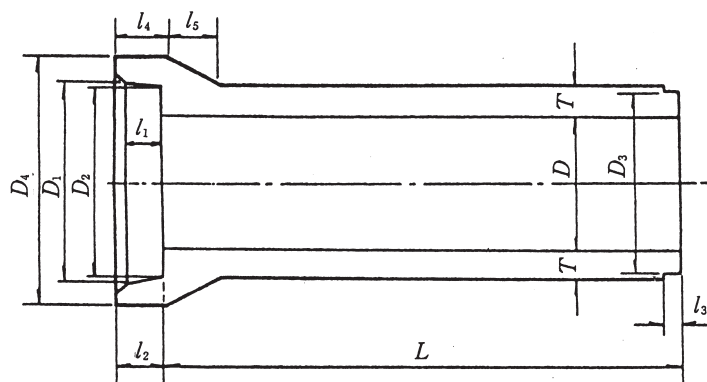
B 形 (JISA5372)
