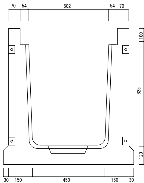
横断側溝 500*600*2000 参考重量 1335 k g
