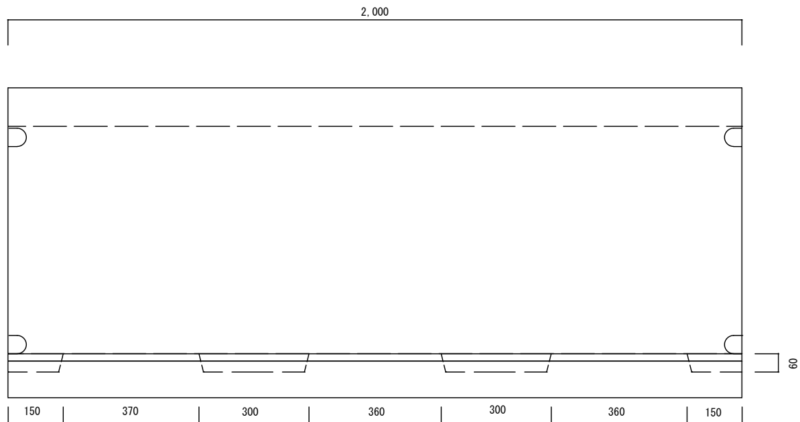
横断側溝 500*600*2000 参考重量 1335 k g
