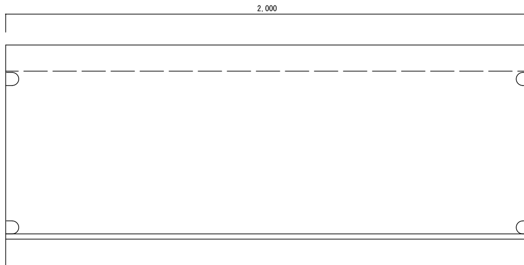
横断側溝 500*600*2000 参考重量 1335 k g
