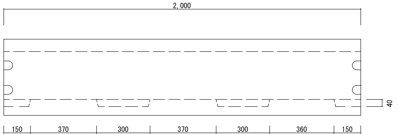
可変横断側溝 GS 250*250*2000 参考重量 508kg
