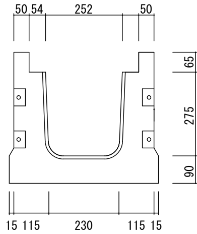
可変横断側溝 GS 250*250*2000 参考重量 508kg
