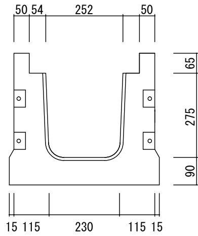
横断側溝 GS 250*250*2000 参考重量 515kg
