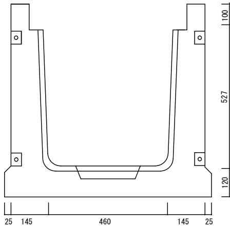
可変横断側溝 500*500*2000 参考重量 1168 k g
