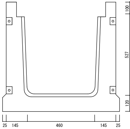
横断側溝 500*500*2000 参考重量 1194 k g
