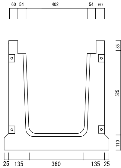
横断側溝 400*500*2000 参考重量 1019 k g
