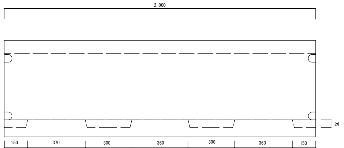
横断側溝 400*500*2000 参考重量 1019 k g
