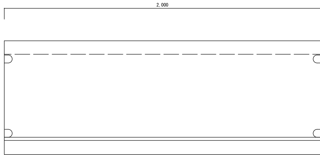
横断側溝 400*500*2000 参考重量 1019 k g
