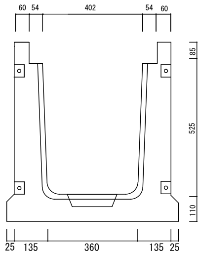
横断側溝 400*500*2000 参考重量 1019 k g
