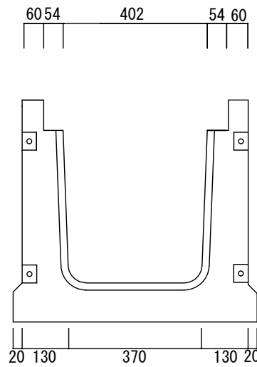
横断側溝 400*400*2000 参考重量 892 k g
