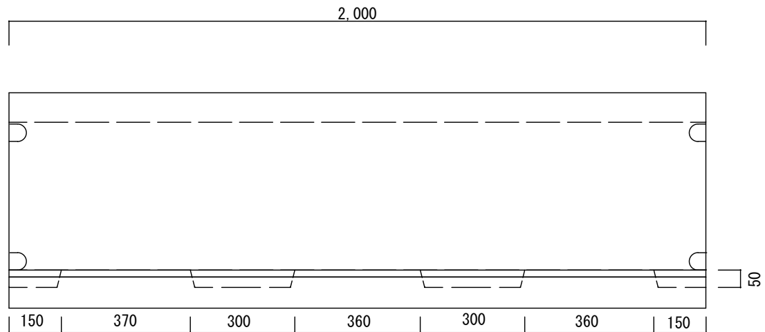
横断側溝 400*400*2000 参考重量 892 k g
