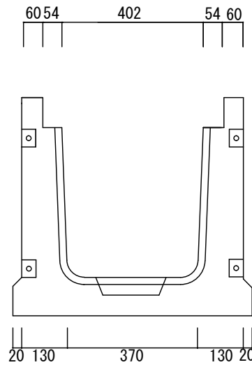
可変横断側溝 400*400*2000 参考重量 876 k g
