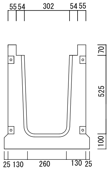
横断側溝 300*500*2000 参考重量 899 k g
