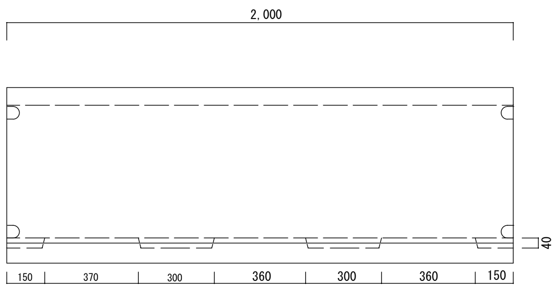
横断側溝 300*500*2000 参考重量 899 k g
