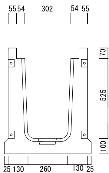
可変横断側溝 300*500*2000 参考重量 892 k g
