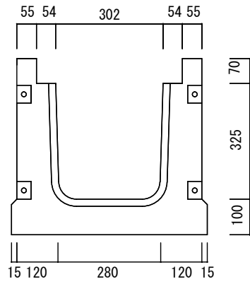
横断側溝 GS 300*300*2000 参考重量 646 k g
