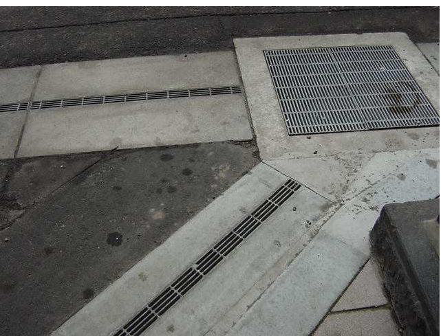
〈コーナー部施工例 2〉
